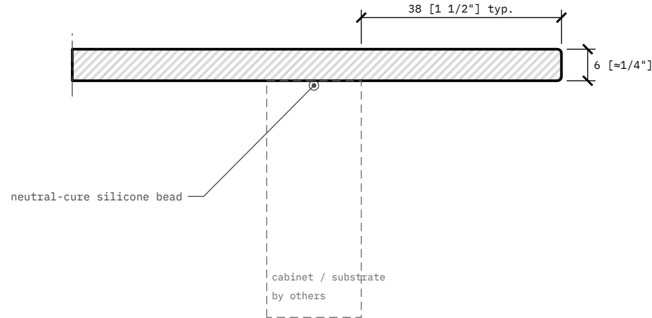
6 D01 6 MM SOLID PLATE SCALE 1:1 · 47.6 kg/m 2 · 9.7 lb/ft 2
